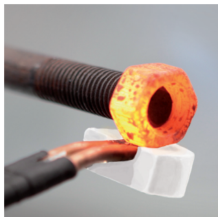
Sprostitev vijakov
